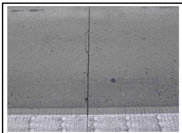
사진번호 70 포장부 S24 줄눈 주변 파손 외관망도 5-10
