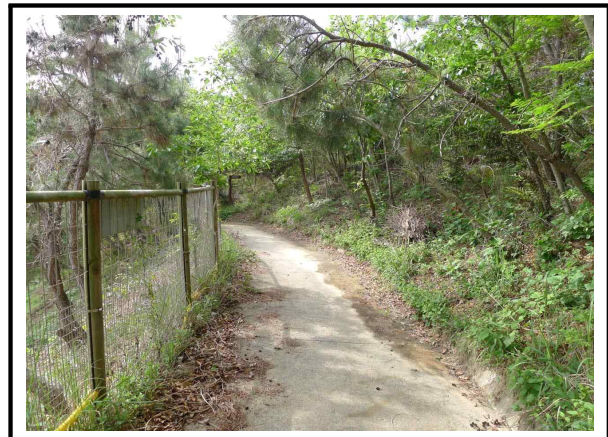
사진번호 82 종점부 사면 소단 배수로 외관망도 -
