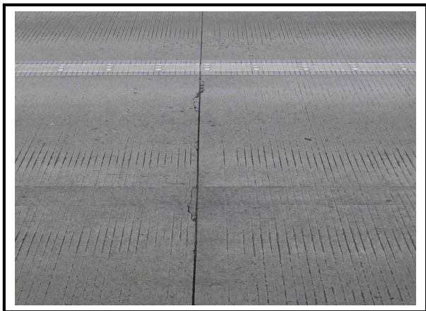
사진번호 67 포장부 S18 줄눈 주변 파손 외관망도 4-6
