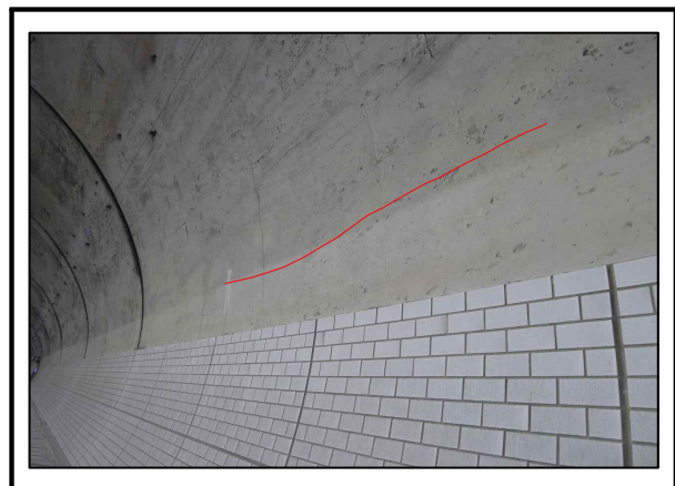
사진번호 34 측벽부 S14 우측 균열(0.3mm미만) 외관망도 3-1
