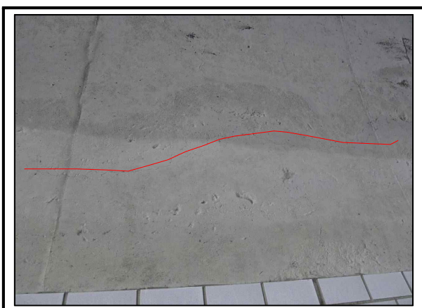
사진번호 35 측벽부 S23 우측 균열(0.3mm미만) 외관망도 5-12
