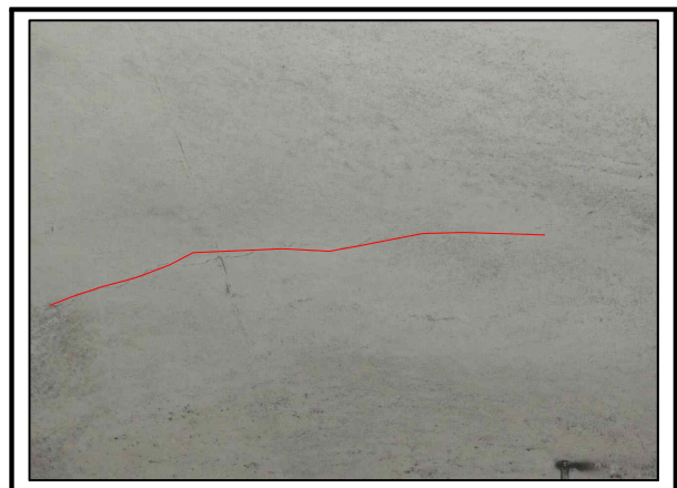
사진번호 22 천단부 S34 외관망도 7-4 균열(0.3mm 이상)
