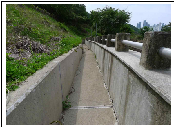
사진번호 81 시점 갱구부 상단 배수로 전경 외관망도 -
